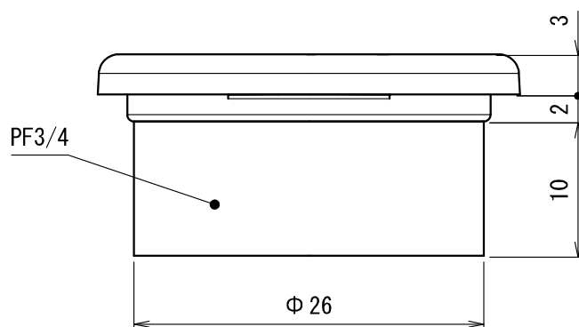
パッキン・ロックナットを外した状態
